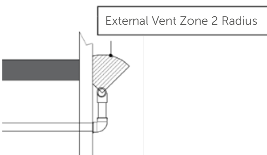
Hyprolyser® 180-8500: Ventilation Zone 2 Radius
